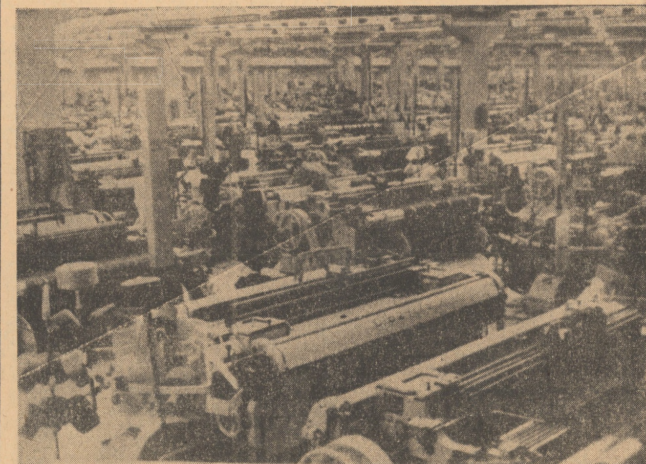
R.P. BULGARIA. Uzina textilă de stat „Dimitar Blagoev” din Kazanluk, una din cele mai moderne din Bulgaria, s-a specializat în confecționarea hainelor din lînă pură și din fibre de polyester. În foto: Vedere generală din hala de țesut a fabricii
