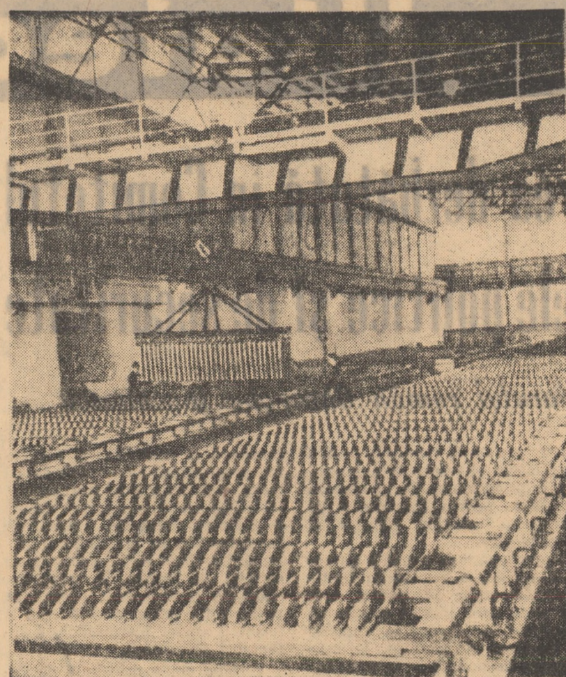
Hala de electroliză a plumbului de la U.C.M. Copșa Mică
