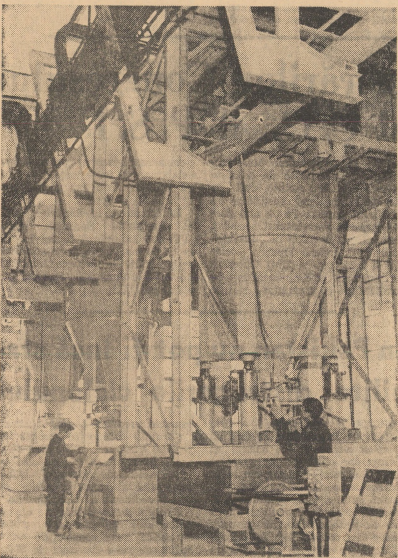
Instalații moderne de fabricare a fritei la uzina „Emailul roșu” Mediaș
