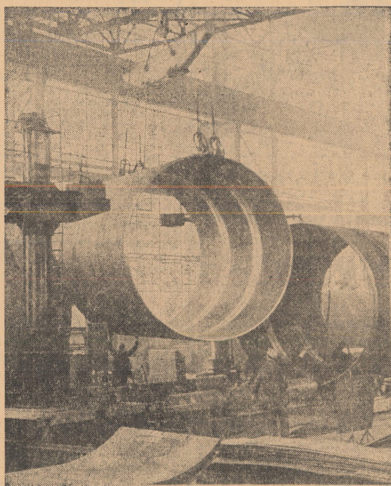
Cazangeria grea a uzinei „Independența” Sibiu — locul unde „se nase” marile virole pentru conducta forțată de la hidrocentrala Lotru
