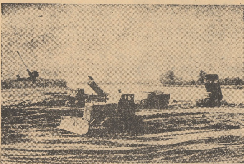
R.S. Cehoslovacă. Cursul riului Vah face o mică curbă în apropiere de satul Kamenica în vecinătatea orașului Komarno (sudul Slovaciei) din care cauză aici au loc dese inundații. Pentru prevenirea acestora, pe această porțiune se schimbă cursul riului pe o lungime de 2.600 m, noua albie avînd o lățime de 150 m și o adîncime de 5 m. Au fost excavate mai mult de 1 milion de tone de pămînt, folosit la construcția stăvilarelor. Prin această lucrare de amploare vor fi redat agriculturii 650 ha. În foto: Lucrări la schimbarea cursului riului Vah
