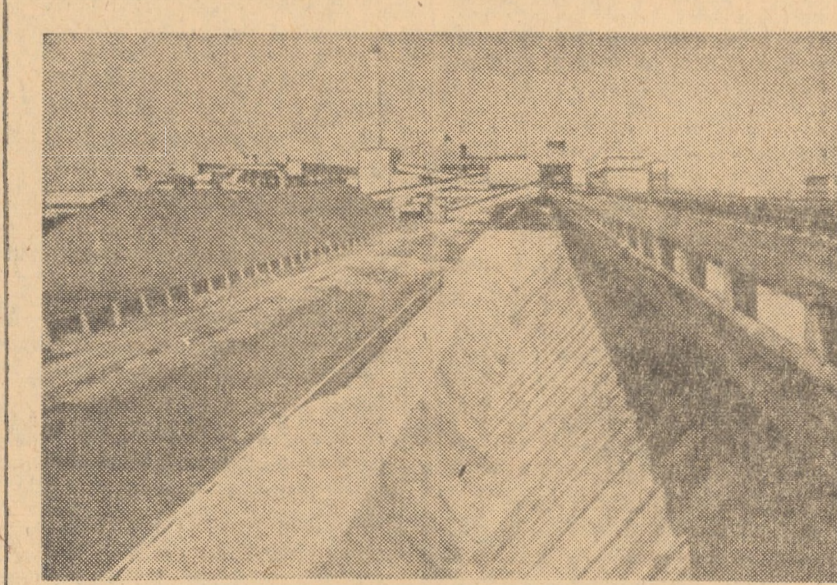
R.P. UNGARĂ. Linie de transport a materialului brut la Uzina de aglomerare a minereului din Sajokeresztur, regiunea Borsod
