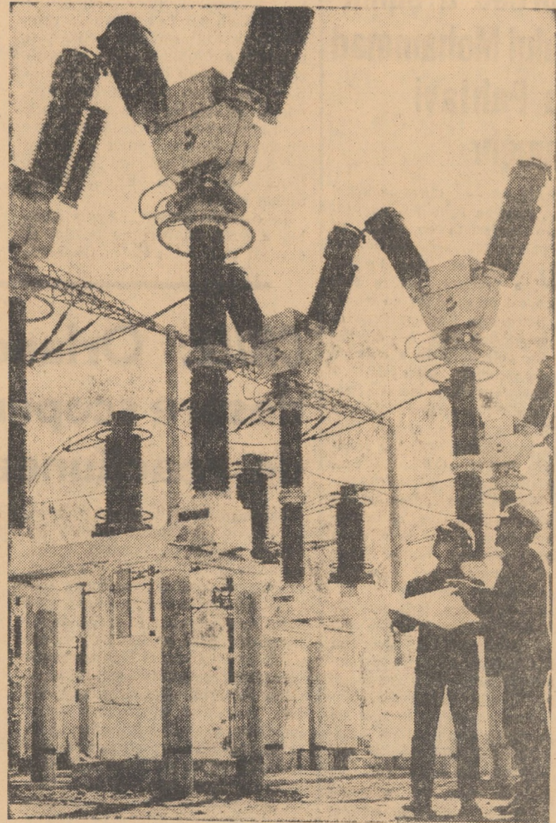
O adevărată „pădure” cu izolatori de înaltă tensiune. (Stația de conexiuni Sibiu)
