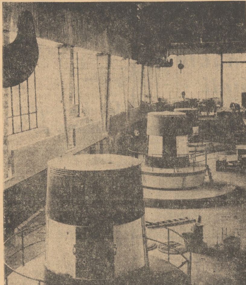
R.P. POLONA. S-au făcut primele probe ale pompelor cu turbine de la noua hidrocentrală de la Zydów. În foto: Sala turbinelor. Capacitatea totală a noii hidrocentrale va fi de 150 MW. Uzina va fi în viitor mărită
