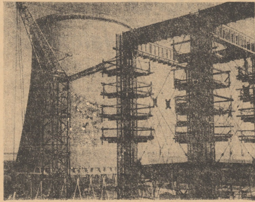
La Viscontia în nordul Ungariei este în construcție termocentrala „Gagarin” în completare, care la ora actuală are o capacitate de 600 MW. Următoarea unitate de 200 MW acum în lucru, va completa capacitatea termocentralei la 800 MW. În foto: turnul de răcire și scheletele noilor construcții
