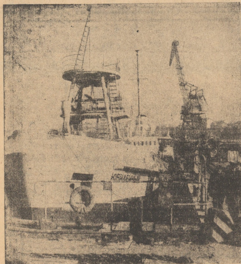
R.P. BULGARIA. În cîstea celui de-al 10-lea Congres al P.C.B., care va avea loc în aprilie, muncitorii șantierului naval „Ivan Dimitrov” din Russe, vor termina un vas de 1.500 tone și vor începe construirea noii serii de petroliere de 5.000 tone destinate exportului. În foto: Vasul de 1.500 tone dat la apă.
