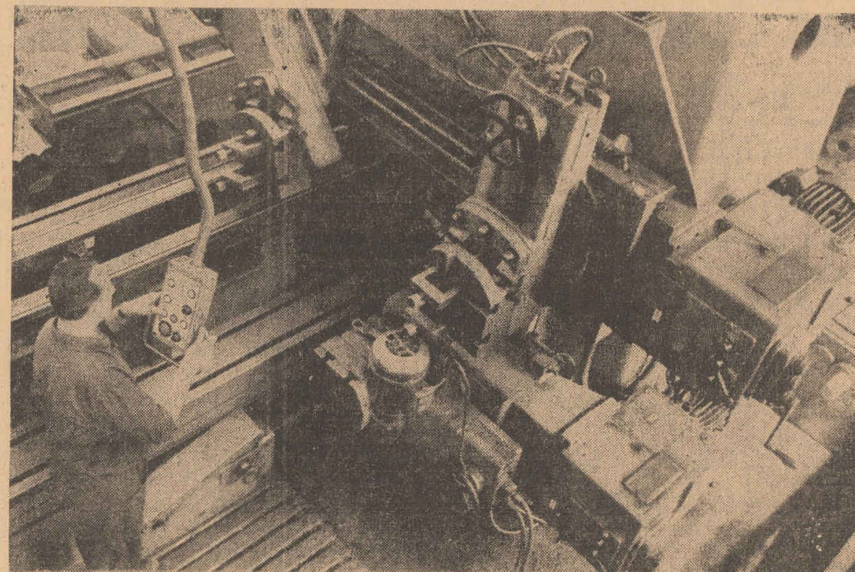
Rectificarea batiurilor strungurilor — operație de precizie — se face în secția uzinaj greu a uzinei „Independența” Sibiu, la o raboteză care figurează printre cele mai mari utilaje prelucrătoare ale uzinei, deservită de comunistul Ion Boeraș
