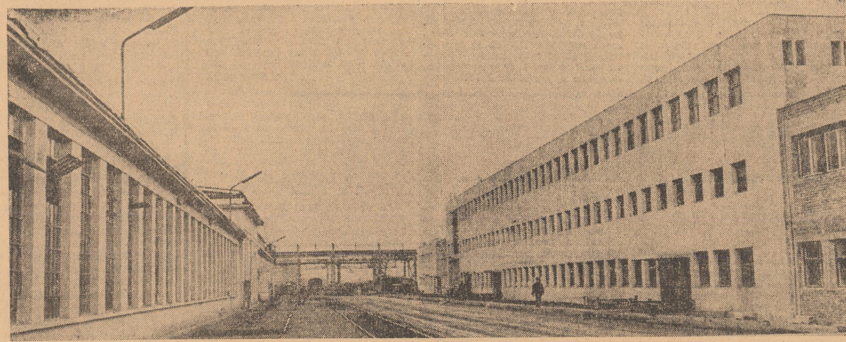
Uzina mecanică Mirsa dispune azi de hale spațioase. În imaginea sculărie și secția de montaj și debitare, construite de-o parte și de alta a unei largi șosele de acces
