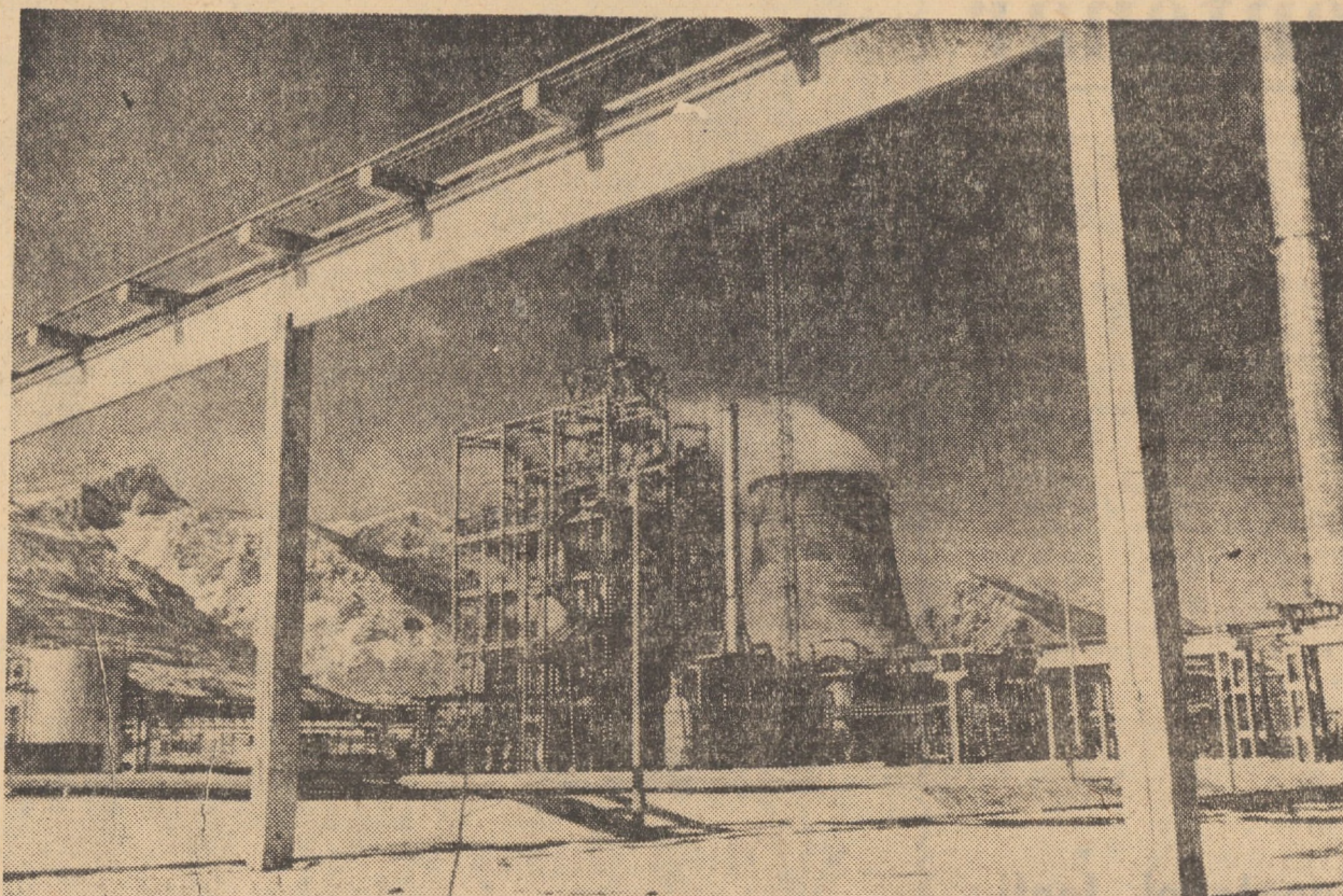
R.P. BULGARIA. La Varna s-a inaugurat noua uzină chimică pentru carbon bisulfat, care va folosi ca materie primă gazul natural. Uzina complet automatizată va produce 20.000 tone de carbon bisulfat, necesar producției de fibre sintetice și în chimie. În foto: vedere a noii uzine chimice din Varna
