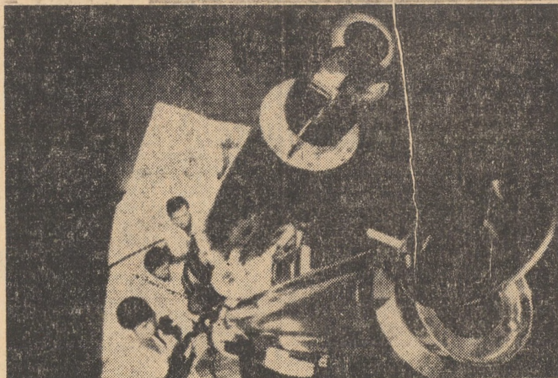
U.R.S.S. R.S.S. Gruzia. Observatorul astronomic din Abasumansk. În foto: Cercetarea Soarelui cu ajutorul dublului telescop, cromosferă-fotosferă
