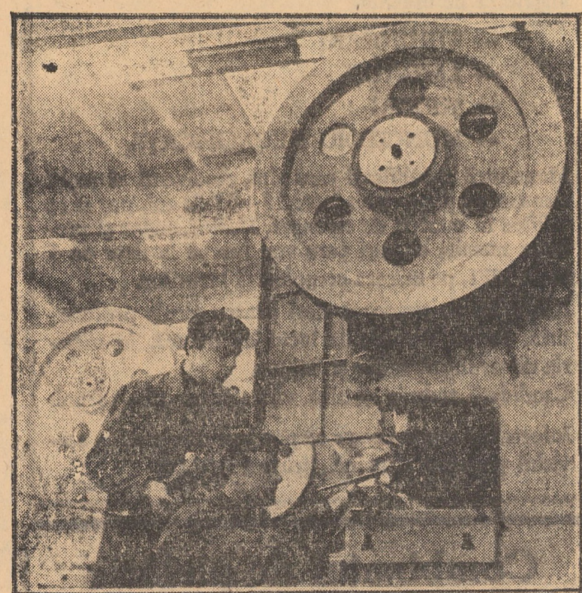
După montaj, înainte de a fi finite, presele cu excentric, produse de Uzina mecanică Sibiu, sînt supuse unui riguros control, verificîndu-se buna funcționare a fiecăreia în parte
