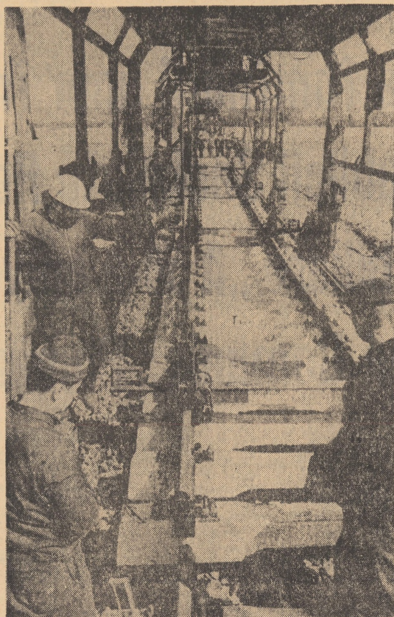
În R.D.G. se află în reconstrucție o porțiune de cale ferată de peste 7 km între Rostock și Stralsund. În foto: după dislocarea secțiunilor din vechia linie, se montează noi secțiuni de linie
