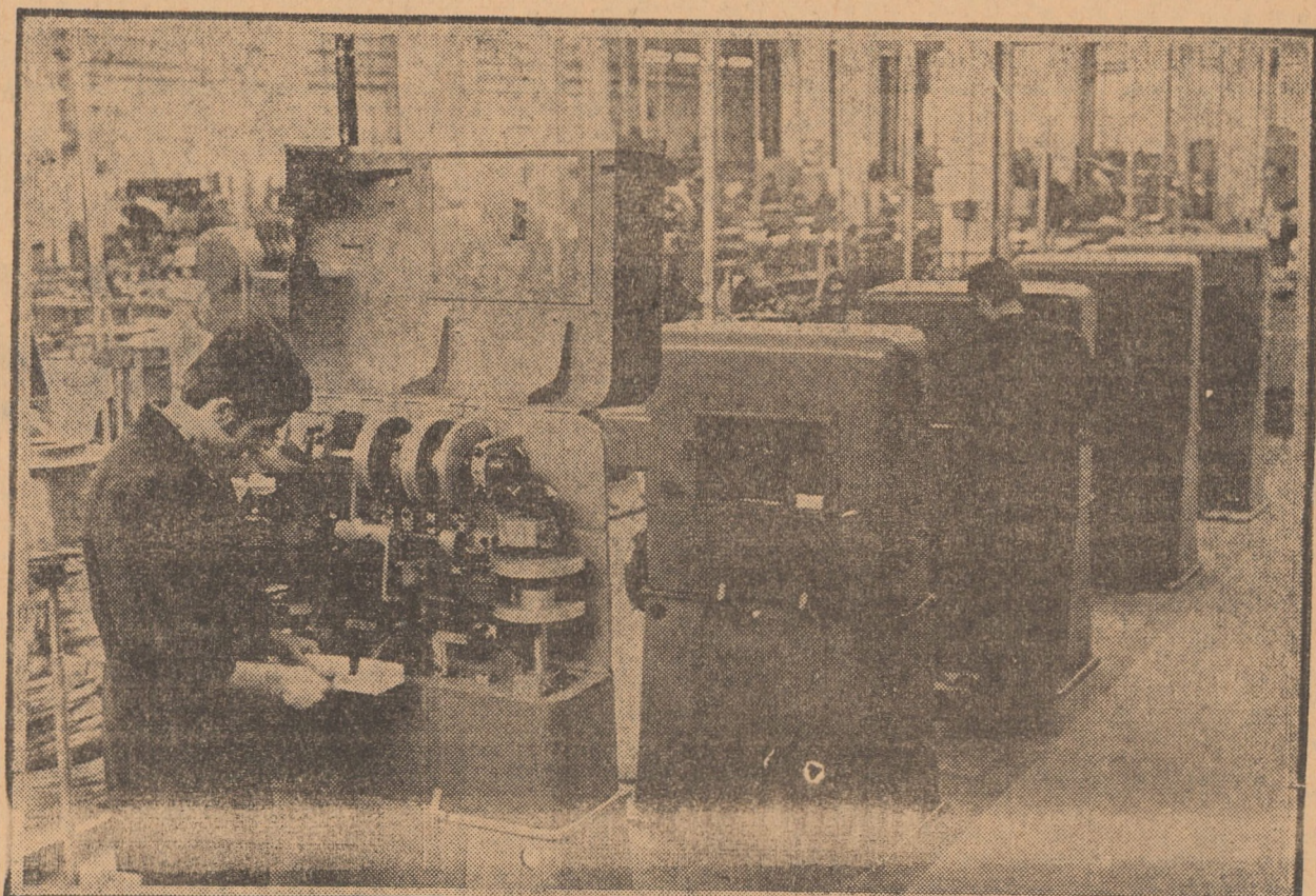
Grupul de mașini automate universale de îndoit sîrmă din secția metal a fabricii „Flamura roșie” Sibiu.
