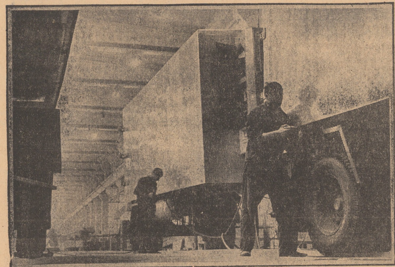
Aspect de la montajul semiremorcilor frigorifice cu instalații proprii de congelare, avînd o capacitate de 37 m.c.m. produsă la uzina „Automecanică” Mediaș
