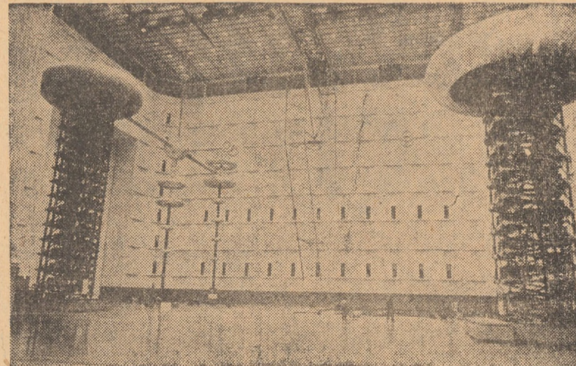
FRANȚA. În curtea Centrului de cercetări EDF „Renardieres” din apropiere de Moret-sur-Loing va aniversa 25 de ani de la înființare. În foto: vedere de ansamblu a laboratorului de încercări de mare tensiune (65x65x45 m înălțime) cu cele două generatoare de șoc care permit experimentarea materialelor de tensiune nominală de 765 kV, ca și elemente de tensiune nominală cuprinse între 1100—1500 kV
