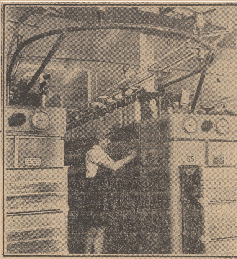
Mașini cu inele de producție românească „Unirea”, utilaje textile moderne cu caracteristici de înaltă tehnicitate, la filatura „11 Iunie” din Cîlnădie
