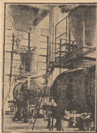
Instalații moderne de fabricare a iritei
