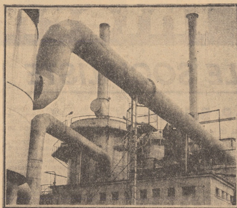
Detaliu din complexele instalații ale U.M.M.N. Copșa Mică
