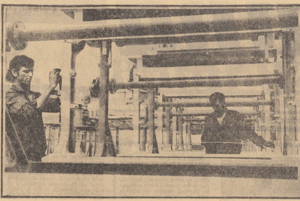
Liviu Nicodin și Traian Burnete, doi dintre lucrătorii atelierului montaj al uzinei „Balansa” Sibiu, executînd ultimele operații de montaj după faza de vopsire la un lot de balanțe automate cu cupă basculantă de 700 kg, folosite la silozuri pentru cîntăritul cerealelor
