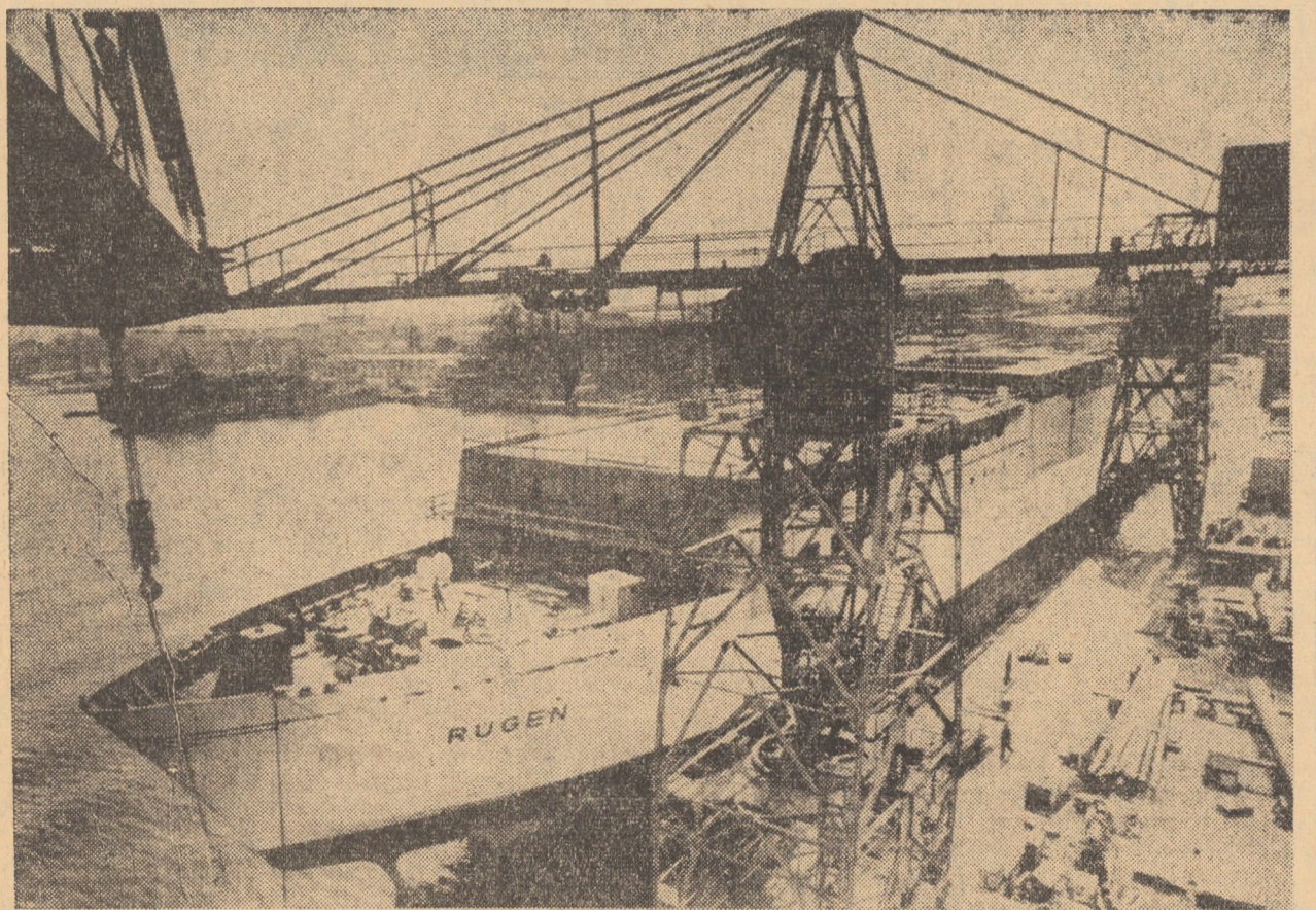
La șantierele navale Neptun din Rostock se află în construcție cel mai mare vas din R.D.G. destinat transportului de vagoane de cale ferată și mașini. Vasul „Rügen“ dispune de o suprafață de 478 m pentru 42 de vagoane și aproape 1.000 m 2 spațiu de parcare pentru camioane și mașini. Vasul are patru motoare de 5.000 C.P. și un deplasament de 6.000 tone. În foto: vasul „Rügen“, în construcție
