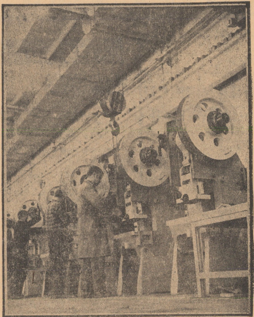
Banda de montaj a preselor automate de 25 tone, produse de Uzina mecanică Sibiu
