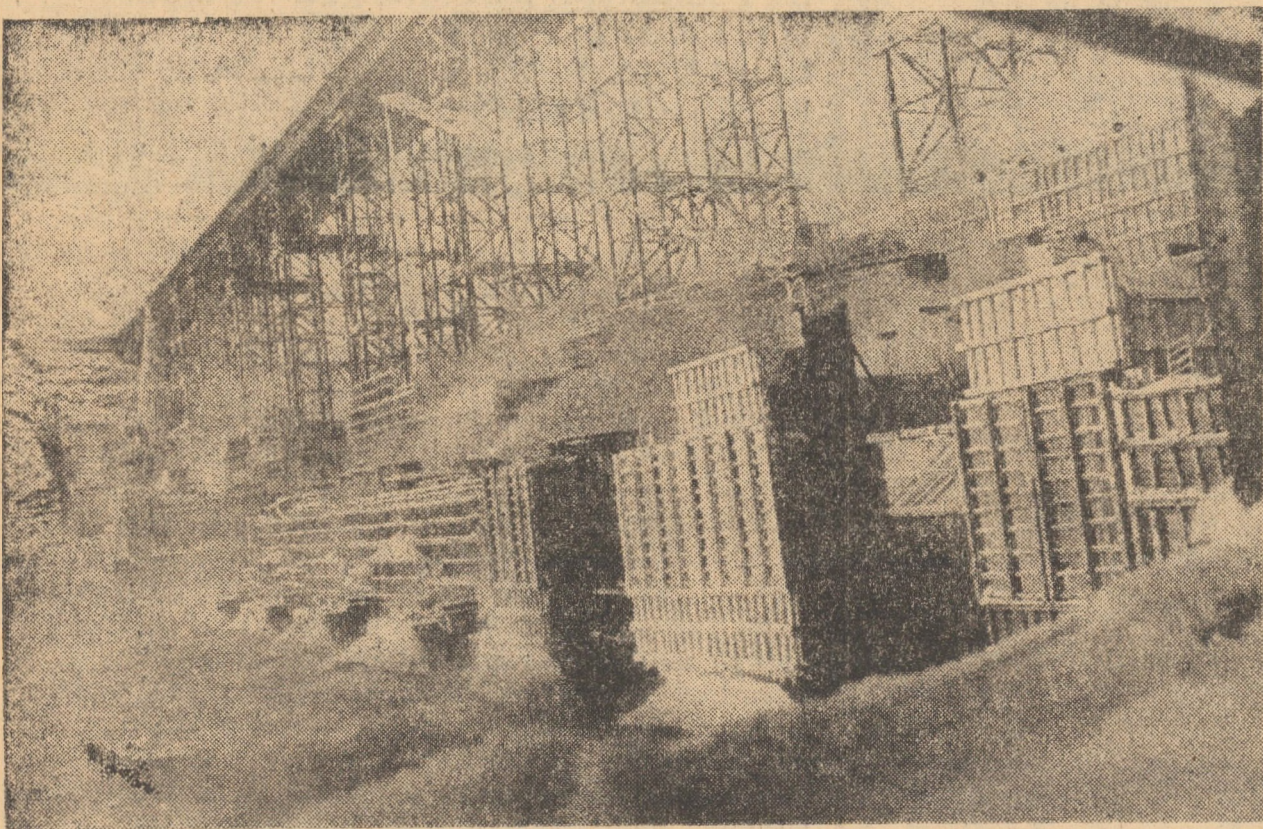
U.R.S.S. Hidrocentrala de pe Angara. Capacitatea proiectată a hidrocentralei Ust-Ilim, care se construiește pe râul siberian Angara, este de 4320000 KW. Aceasta este cea de-a treia hidrocentrală din cascada de pe Angara. În anul 1974 vor intra în funcțiune primele din cele 18 agregate ale acestui obiectiv. În prezent lucrările de construcție sînt în toi. De remarcat că în timpul lucrărilor constructorii intervin cu corective în proiectul inițial în vederea ridicării calității construcției, scăderii prețului de cost. În foto: Pe șantiierul hidrocentralei
