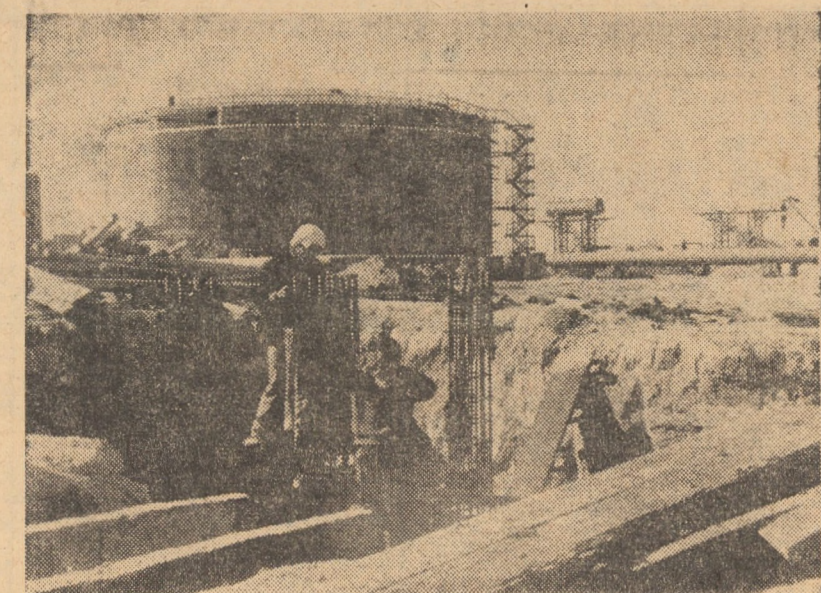
IRAK. În cadrul primei etape de creare a unei industrii petroliere proprii în Rumaila de Nord (Irak) se construiește prima rafinărie națională de petrol. Din Rumaila petroliul va călători cu o conductă specială până în portul FAO. În foto: Pe șantierul viitoarei rafinării
