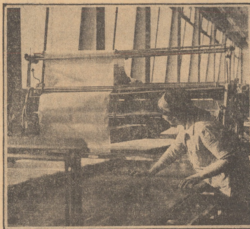
Mașină modernă de spănit (tesături diferite, folosită în procesul productiv la Fabrica de confecții Sibiu)
