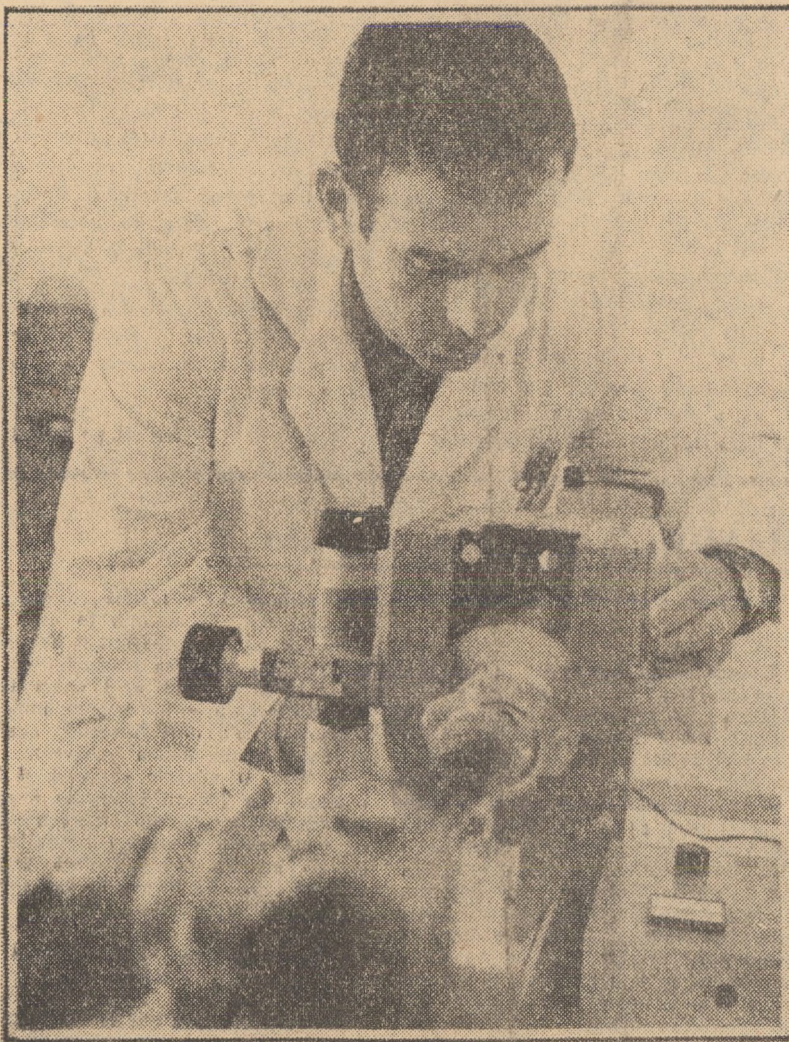
Ing. chimist Eugen Jimon, de la Laboratorul de Cercetări al uzinei „Emailul roșu” Medias, efectund — cu ajutorul unui microscop cu încălzire — determinări ale constantelor emailurilor, în vederea elaborării rețetei.
