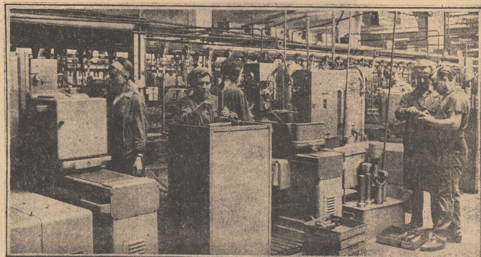
Linie modernă cu mașini de rectificat — canelurile pentru axe cardan la U.P.A. Sibiul
