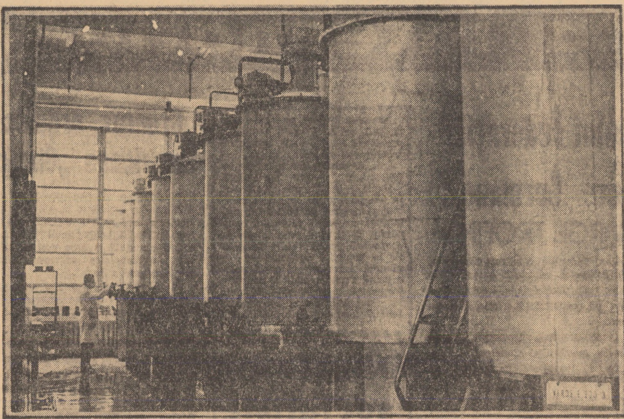
Recipienți pentru captarea emailurilor la uzina „Emailul roșu” Mediaș
