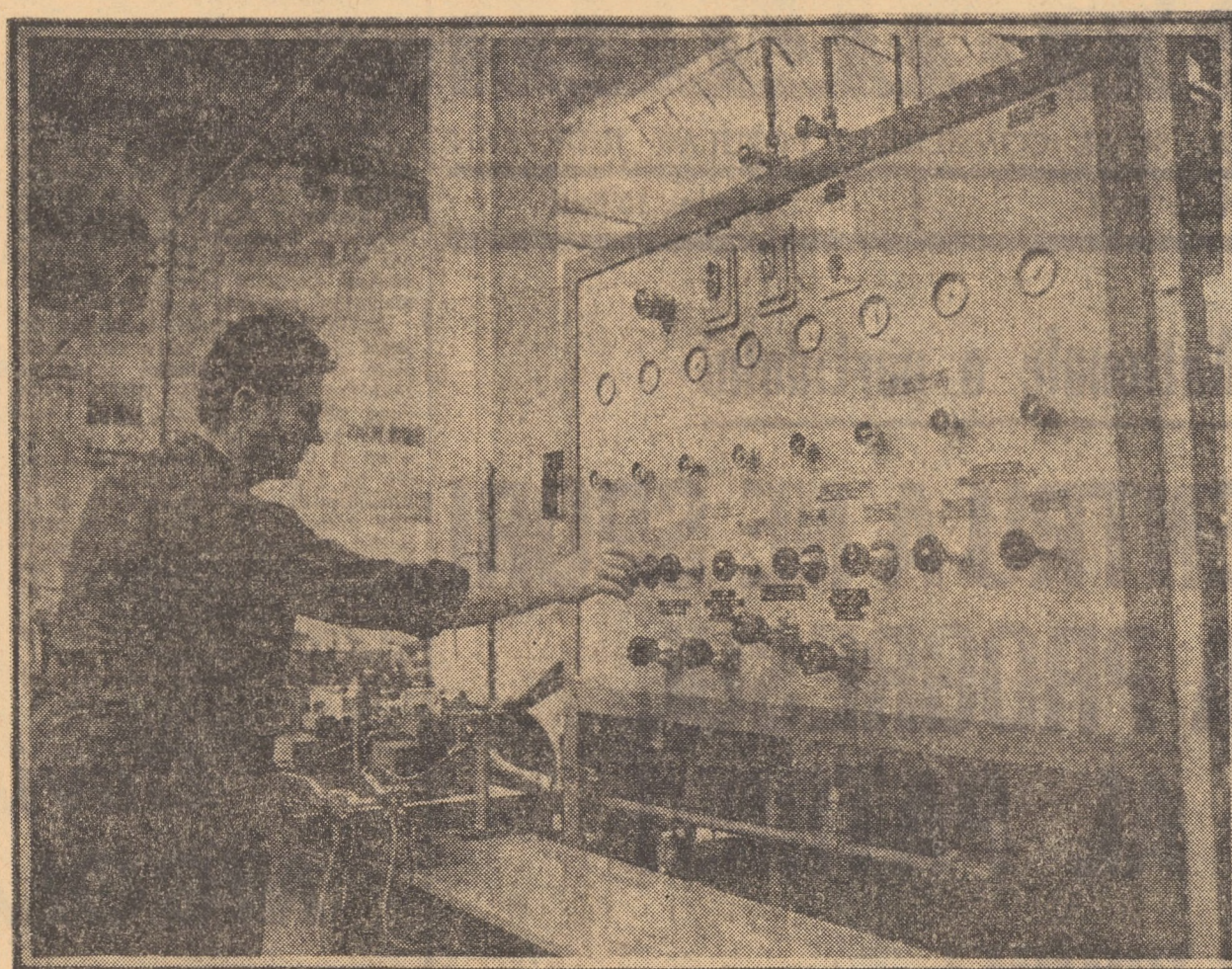
Instalația modernă de tratament termic a garniturilor rigide, complet automatizată, de la „Flaro” Sibiu. În fotografie: tabloul de comandă pentru reglarea debitului de gaze și oxigen, necesar procesului de călire
