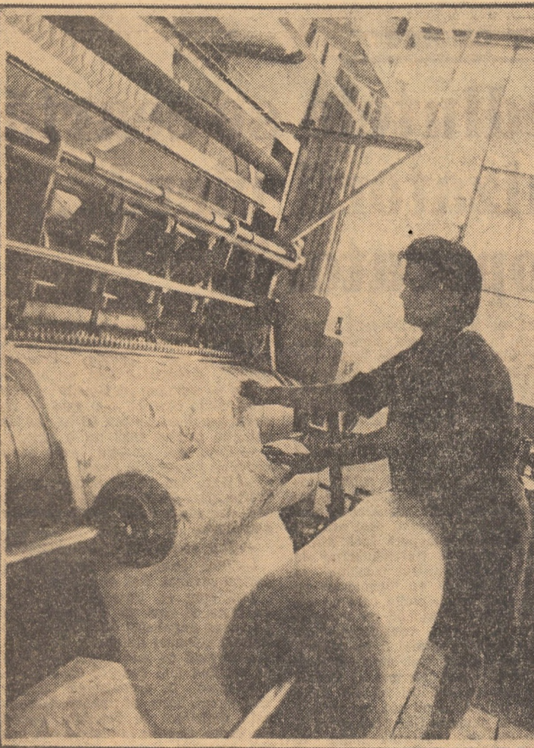
Una din mașinile moderne de mătase țesături de la fabrica „Mătasea roșie” Cisnădie, a cărei productivitate se ridică la cca. 200 m.l. țesături în 8 ore, realizîndu-se diferite modele de cusături
