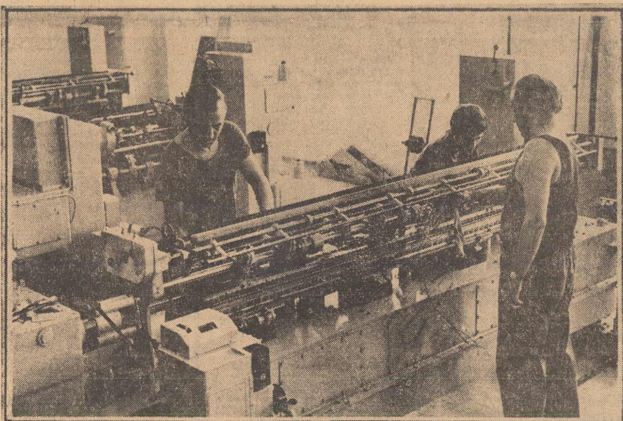
Montarea mașinilor rapide de tricotat urzeală într-una din halele noi ale construcției industriale a fabricii „Drapelul roșu” Sibiu.
