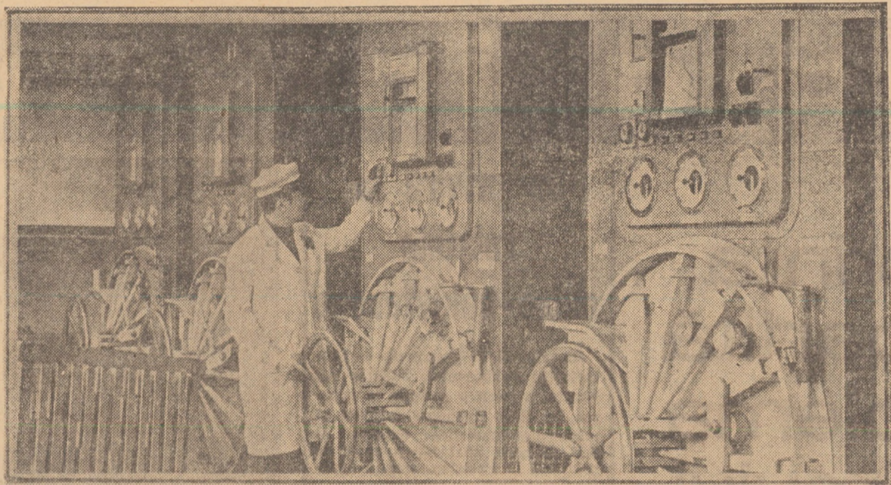
Rotoclave — instalații moderne de sterilizare a preparatelor din carne în cadrul fluxului tehnologic de la F.P.C.C. Sibiu
