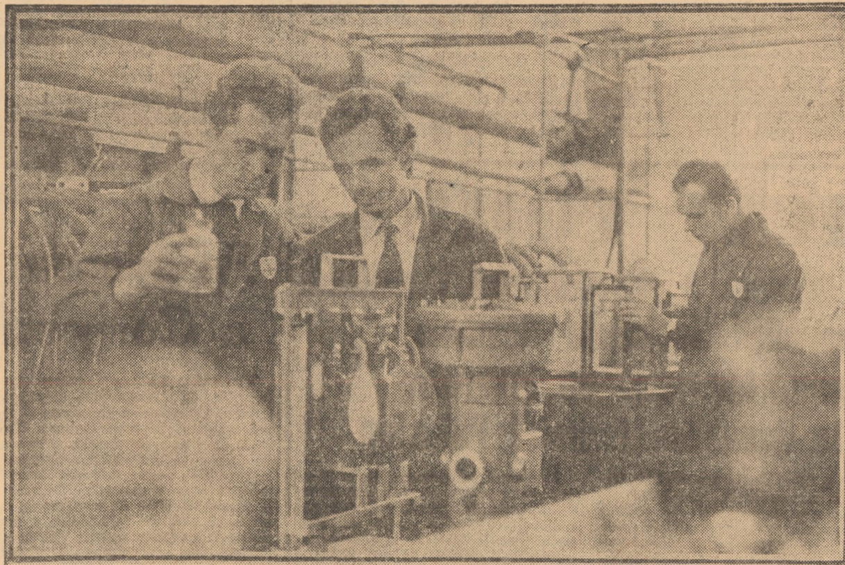
Laborator termotehnic al centrului de cercetare din cadrul Centralei industriale gaz metan Mediaș. Stabilirea parametrilor unui arzător cu aer insuflat de la uzina „Metrom” Brașov. În foto: ing. Octavian Velicea, Reinhold Bielz — tehnician, ing. Iuliu Fodor
