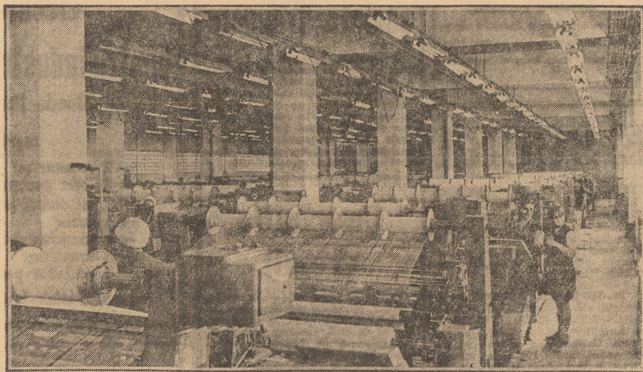
„Drapelul roșu” — unitatea a II-a Sibiu. Aspect din secția mașini rapide de tricotat cu urzeală
