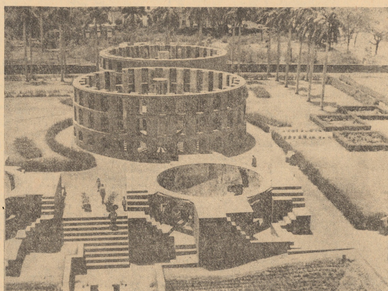
INDIA. În foto: Vedere a Observatorului Astronomic „Jantar Mantar” (Instrumentele Magice) înălțat de regele astronom Maharajah Jai Singh al doilea din Jaipur, care obișnuia ca de aici să privească corpurile cerești.
