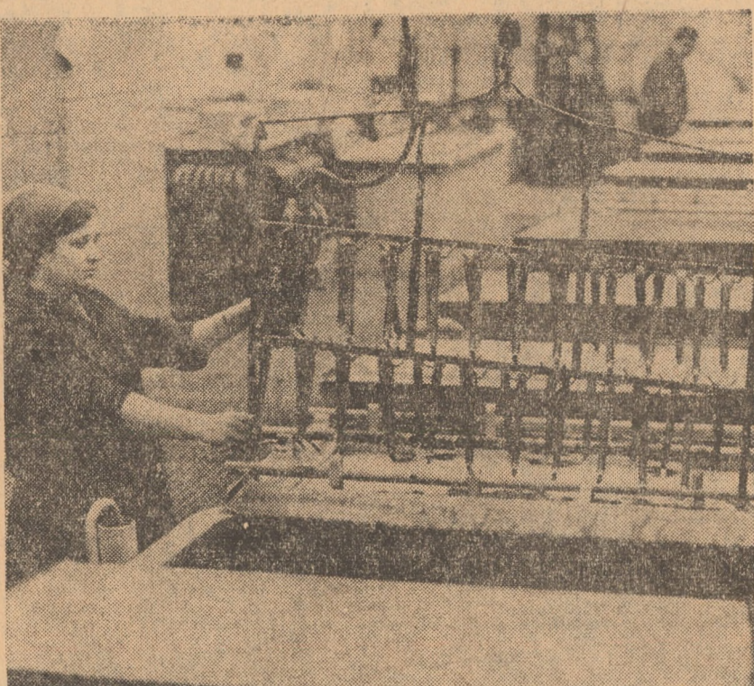
În secția acoperirii galvanice a uzinei „Balanta” din Sibiu, utilaje moderne de mare randament asigură realizarea unor repere de calitate, necesare produselor executate aici
