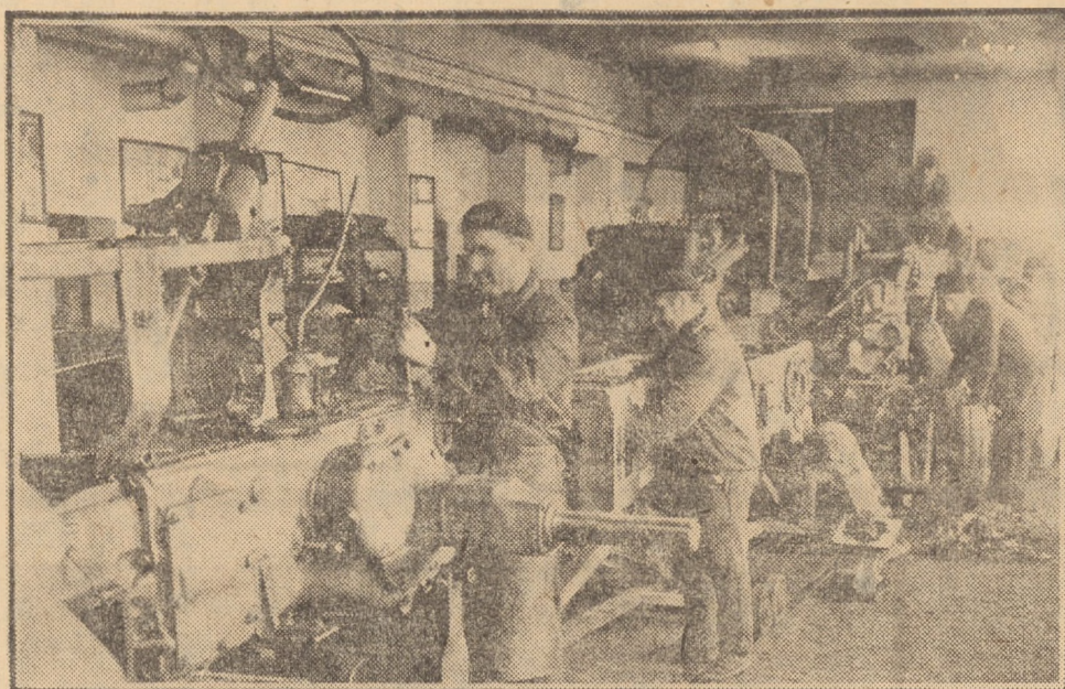
Centrul de reparații S.M.A. Sibiu. Ultimele din cele 32 tractoare, la care se execută reparații capitale, vor fi terminate înainte de termen, cu câteva zile. În fotografie: banda de montaj din atelierul de reparații.
