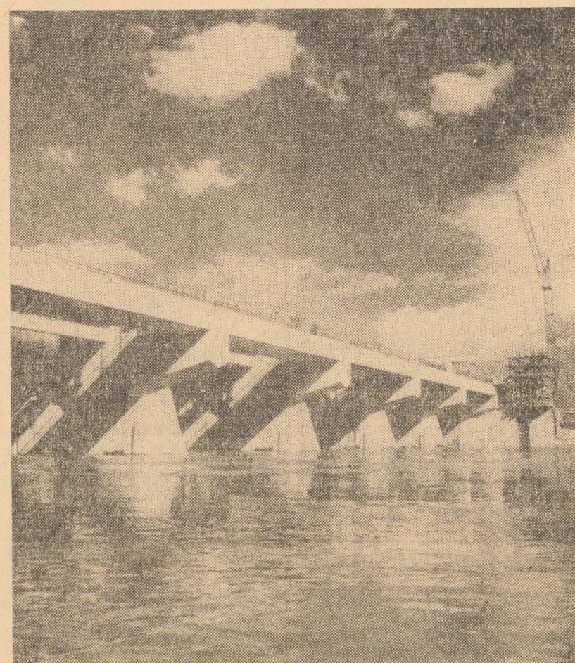
R. P. UNGARĂ. — Vedere parțială a Barajului nr. 2 de pe Tisa, aflat în construcție
