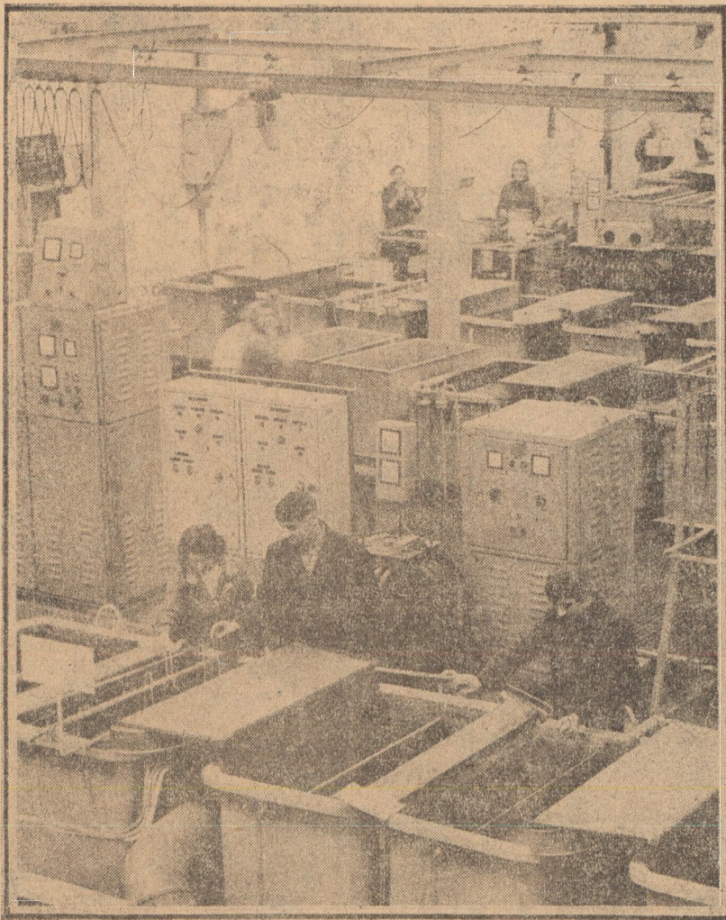
Cerintele tot mai crescînde ale calității produselor, realizate la uzina „Balanta” Sibiu, au impus introducerea de utilaje moderne, perfecționate, cum sînt cele din secția acoperiri galvanice (moderne, perfecționate, cum sînt cele din secția acoperiri galvanice)
