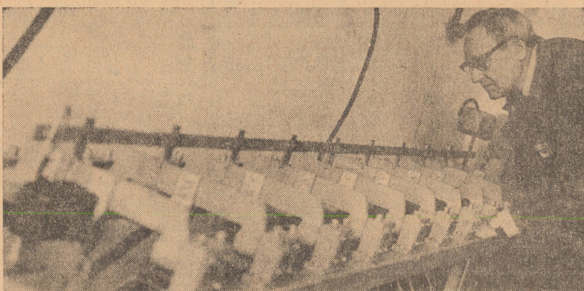
În vederea stabilirii gradului de uzură a pernărilor din tablă, folosite la aparatele de cîntărit, la uzina „Balanta“ din Sibiu a fost realizat, recent, un stand de probă, amplasat în laboratorul de fiabilitate.
