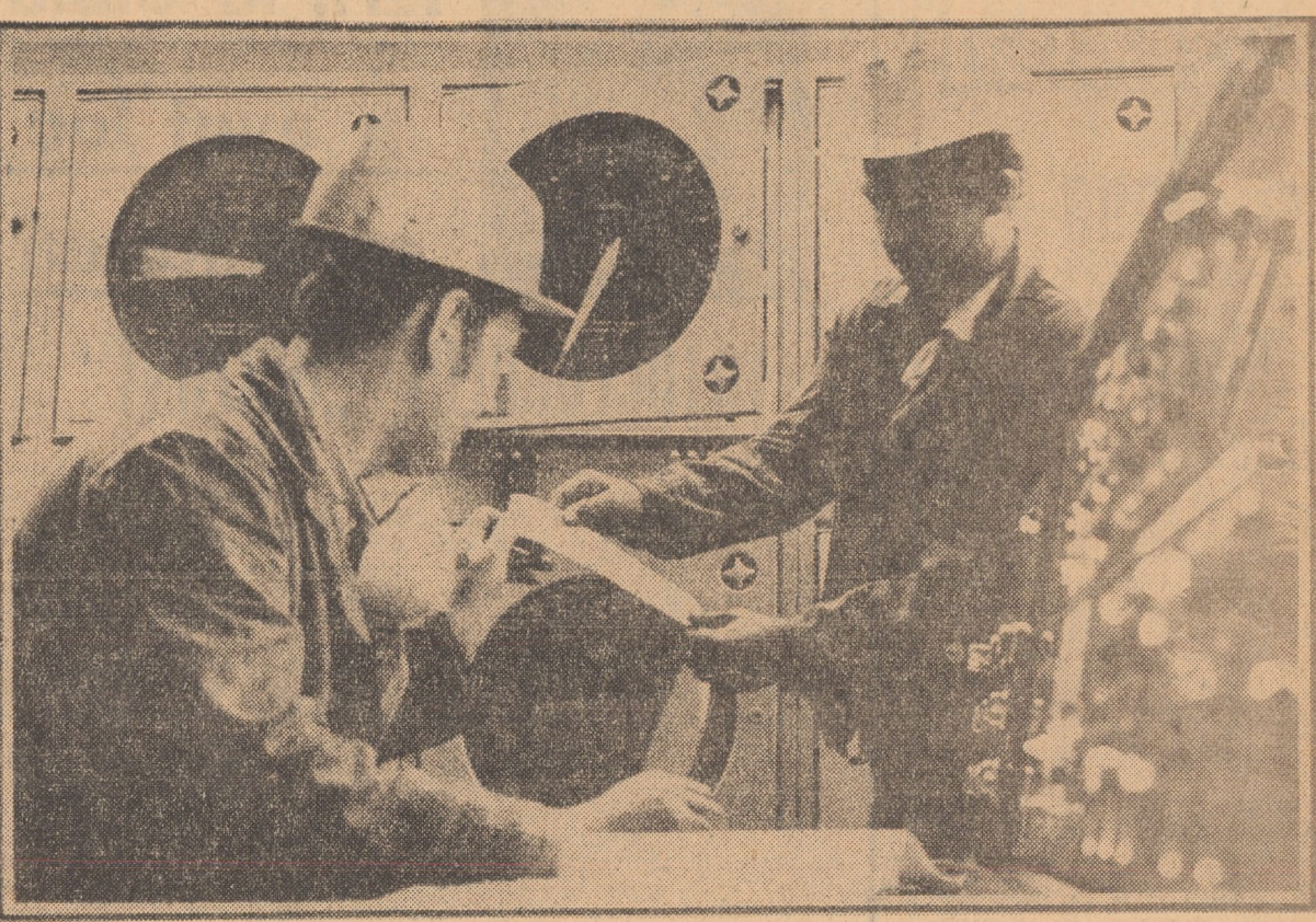
La U.M.M.N. din Copșa Mică, furnul este supus de oameni unor continue transformări care vizează mărirea capacității de producție. Mărirea vitezei de însuflare a aerului, amplificarea hornurilor condensatorilor și alte modificări gândite și realizate de inginerii, maistrii și muncitorii de înaltă calificare au determinat de acum un spor de capacități de peste 50 la sută. În prezent se fac intense pregătiri pentru aplicarea unei noi perfecționări tehnice - schimbarea sistemului de răcire cu apă - prin care se vor cucerii alte sporuri de producție. Fotografia de față vă redă un aspect din camera de comandă a secțiunii de șarjare a furnului Foto: FRED NUSS
