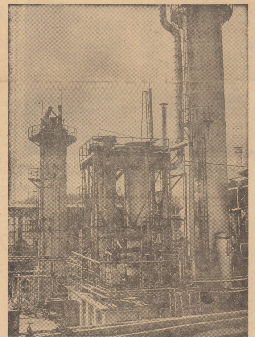
Combinatul chimic Victoria, instalația de formol II
