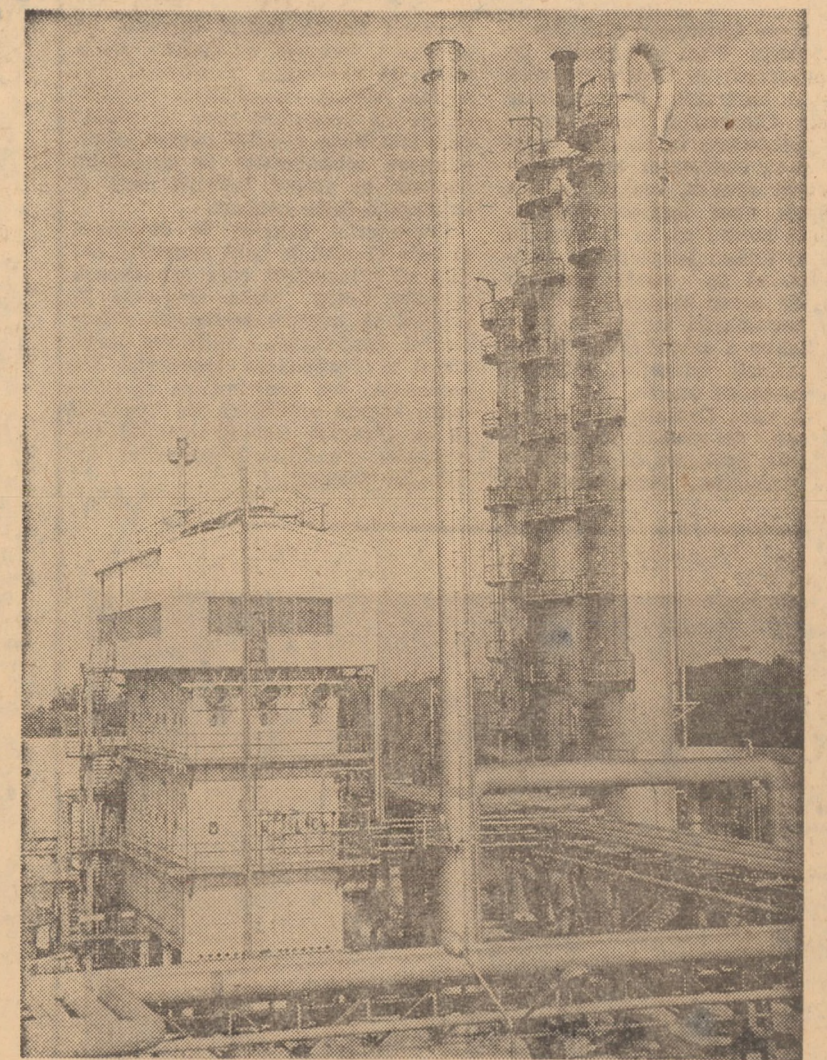
Instalația de cracare și turnurile pentru spălarea bioxidului de carbon
