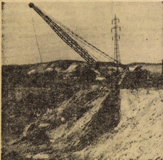
Utilaje de mare capacitate, lucrînd la regularizarea cursurilor de apă
