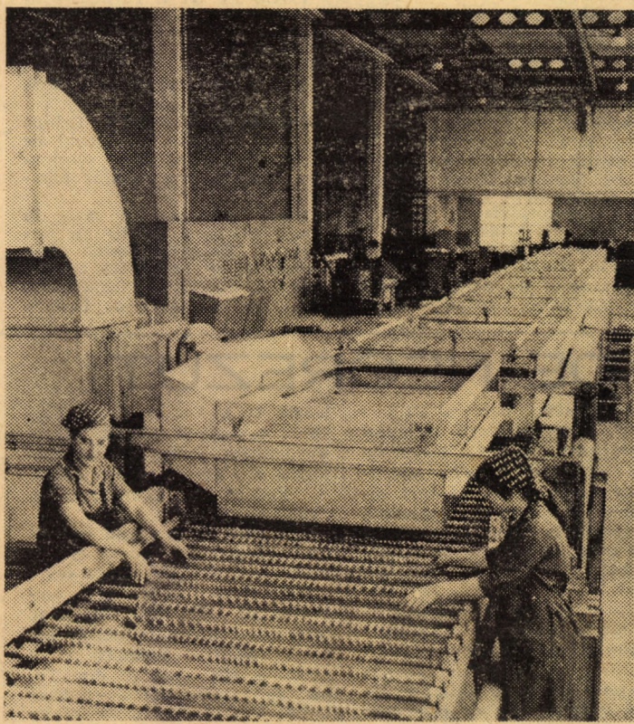
Fabrica de geamuri Mediaș. Linia de securizare orizontală
