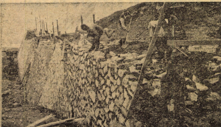
Una din construcțiile destinate protecției Transfăgărășanului: zid de deviere a avalanșelor
