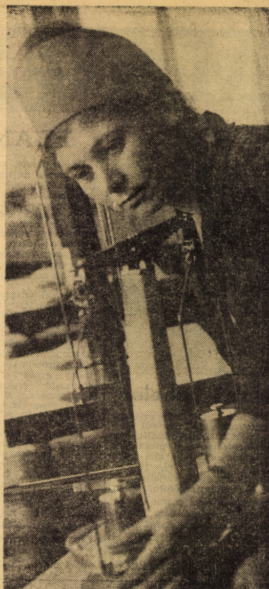
Întreprinderea „Balanța” Sibiu. Montarea și verificarea balanțelor analitice de 1 kg, folosite în laboratoare — operație cu un înalt grad de dificultate — este efectuată de Margareta Schuster, lăcătuș cu o bună pregătire profesională
