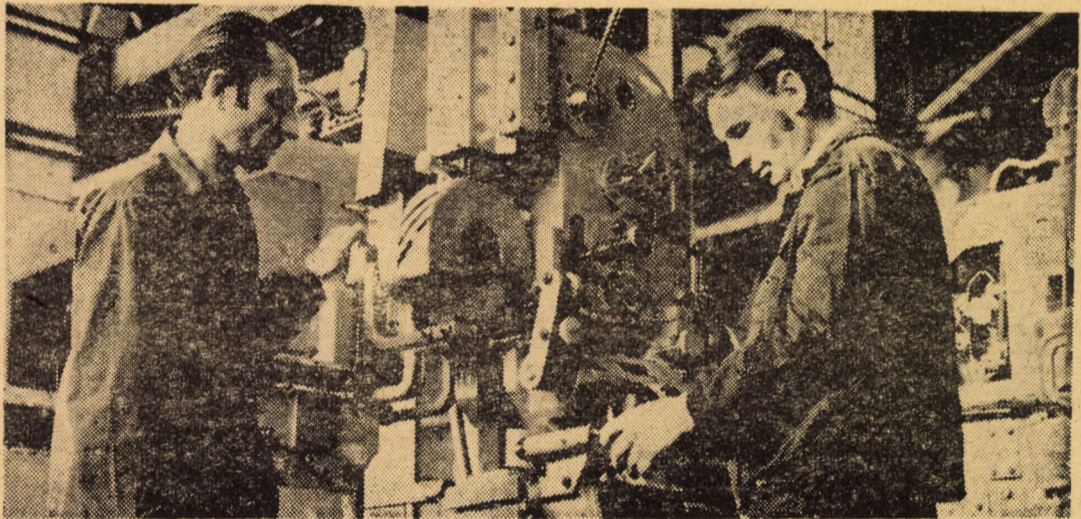
I.U.P.S. Sibiu. Secția utilaje — piese schimb. Finisarea unui grup de mașini automate de ascuțit pinză fierăstraie cu 3 profile de dinți destinate industriei lemnului
