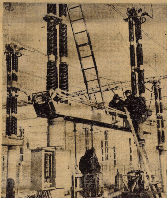
Stația 400 kV Sibiu-sud. Revizia unui intrerupător de 400 kV, la una din celele de linii
