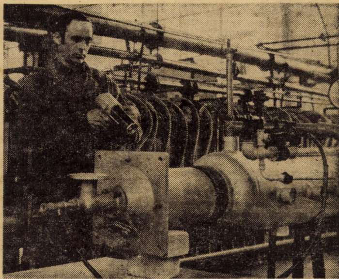
Verificarea condițiilor de ardere a arzătoarelor cu impuls în laboratorul de cercetare a produselor de la Uzina mecanică gaz metan Mediaș Foto: HORST BUCHFELNER
