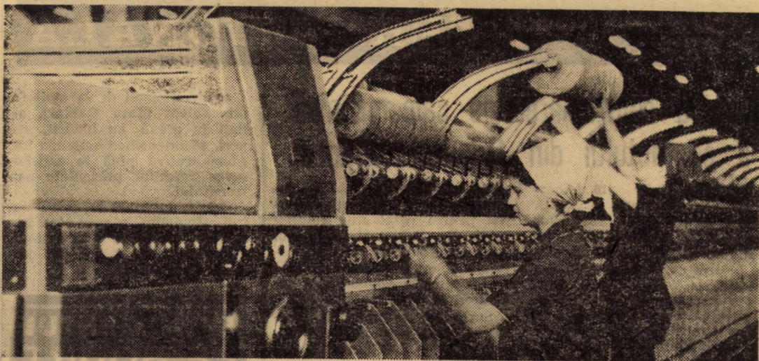
Aspect din secția filatură a I.S. „Textila” Cisnădie. Mașina tip „Unirea” de fabricație românească, realizată la parametrii tehnicii mondiale, completează zestrea tehnică a întreprinderii
