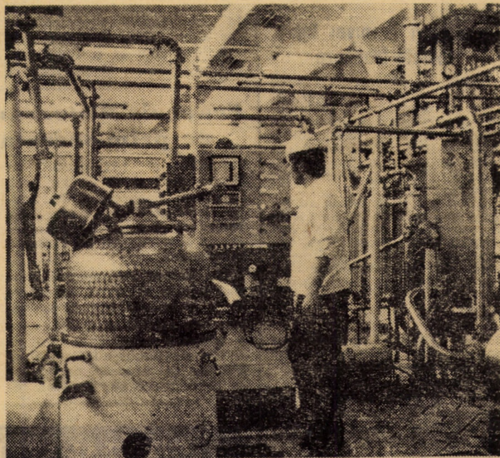
Întreprinderea de industrializare a laptelui Sibiu. Instalația de pasteurizare a laptelui cu o capacitate de 10.000 litri pe oră
